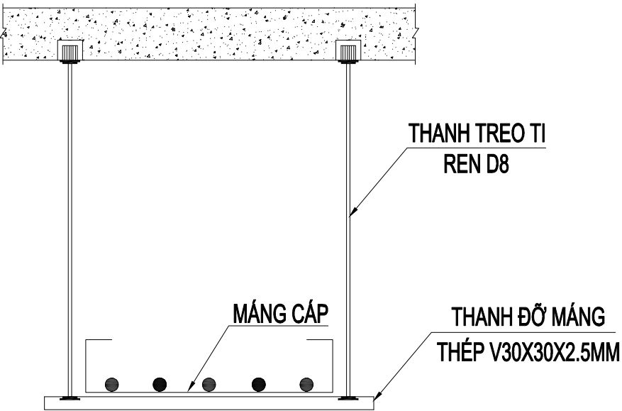
CHI TIẾT LẮP ĐẶT MÁNG
