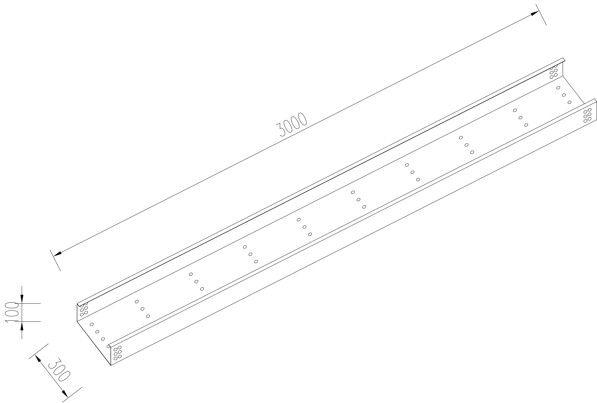
CHI TIẾT MÁNG CÁP
